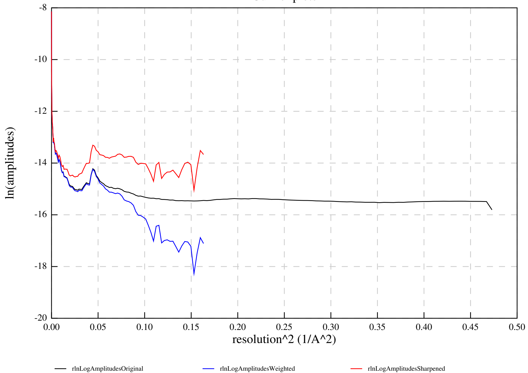
Guinier plots
