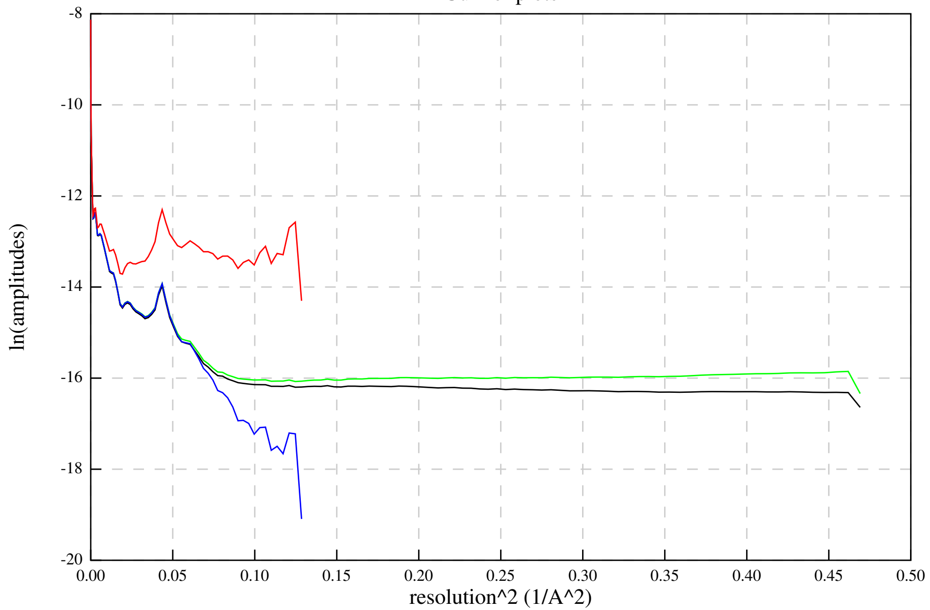
Guinier plots
