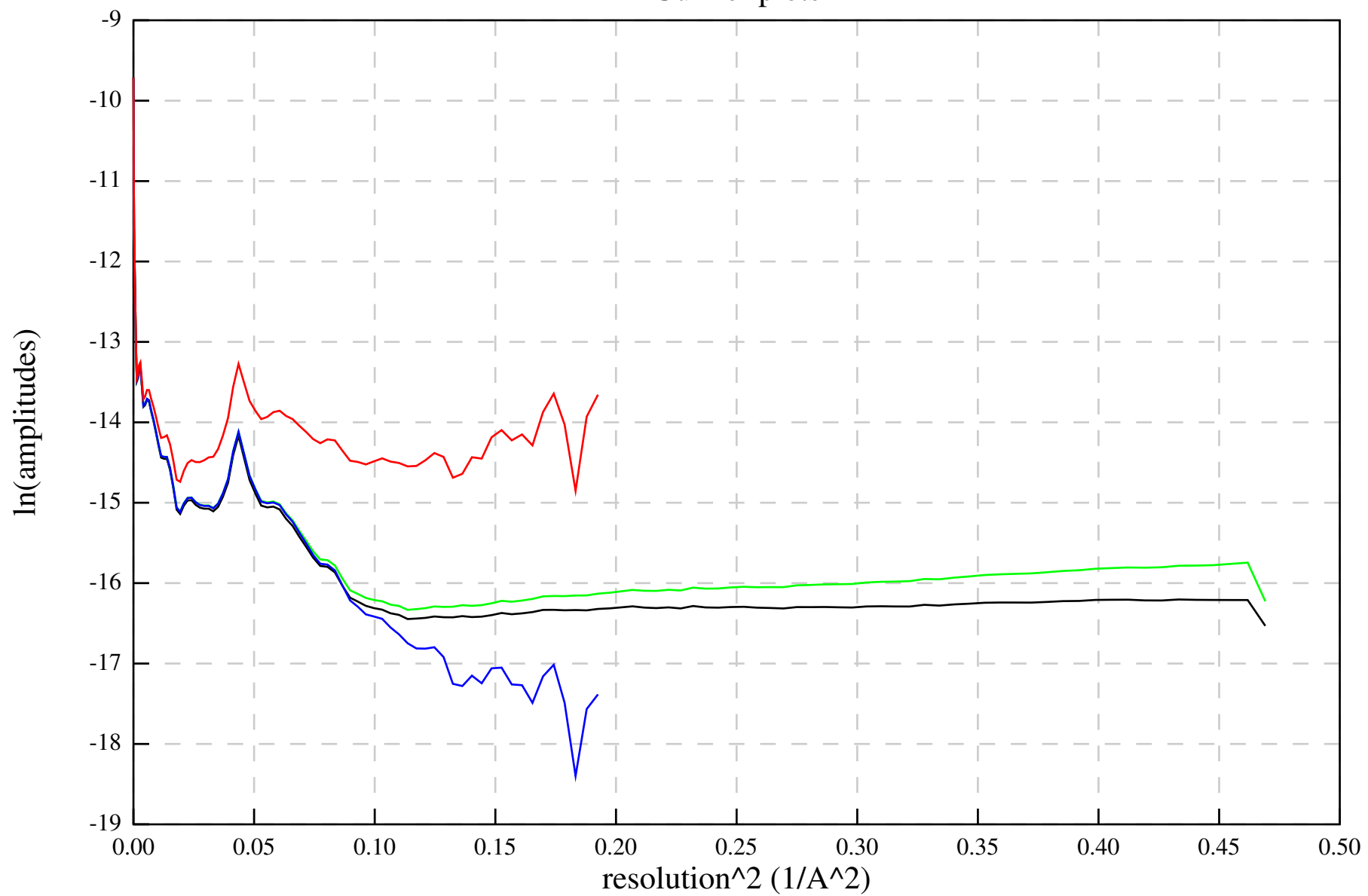
Guinier plots
