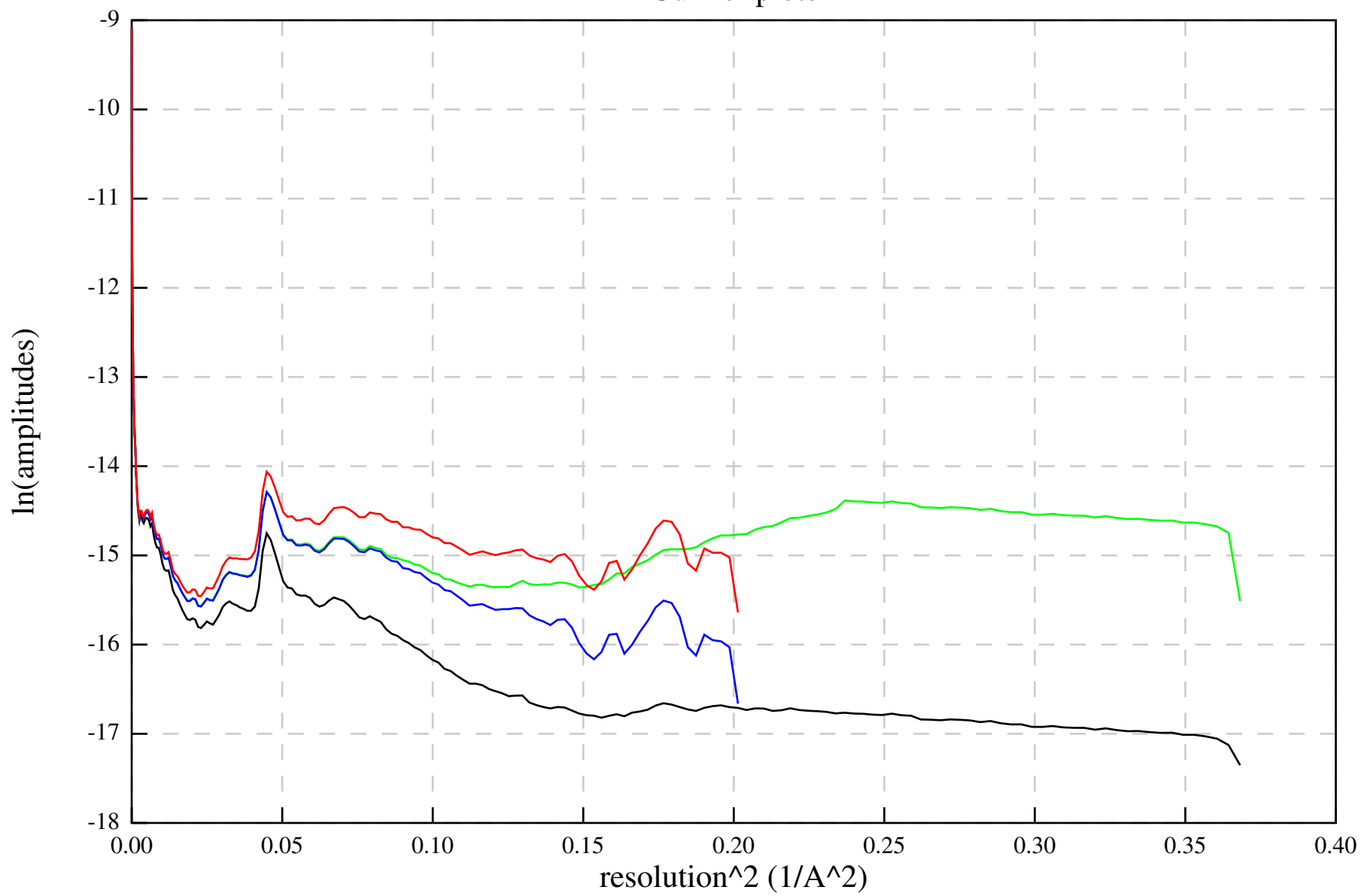
Guinier plots
