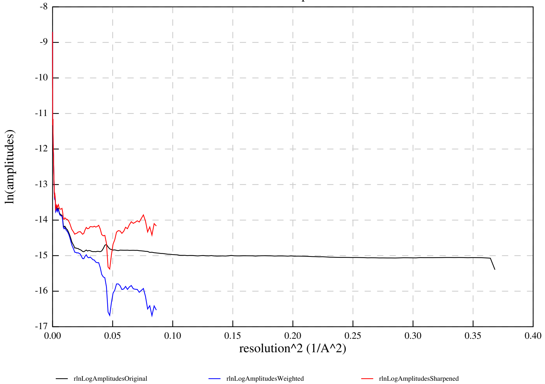
Guinier plots
