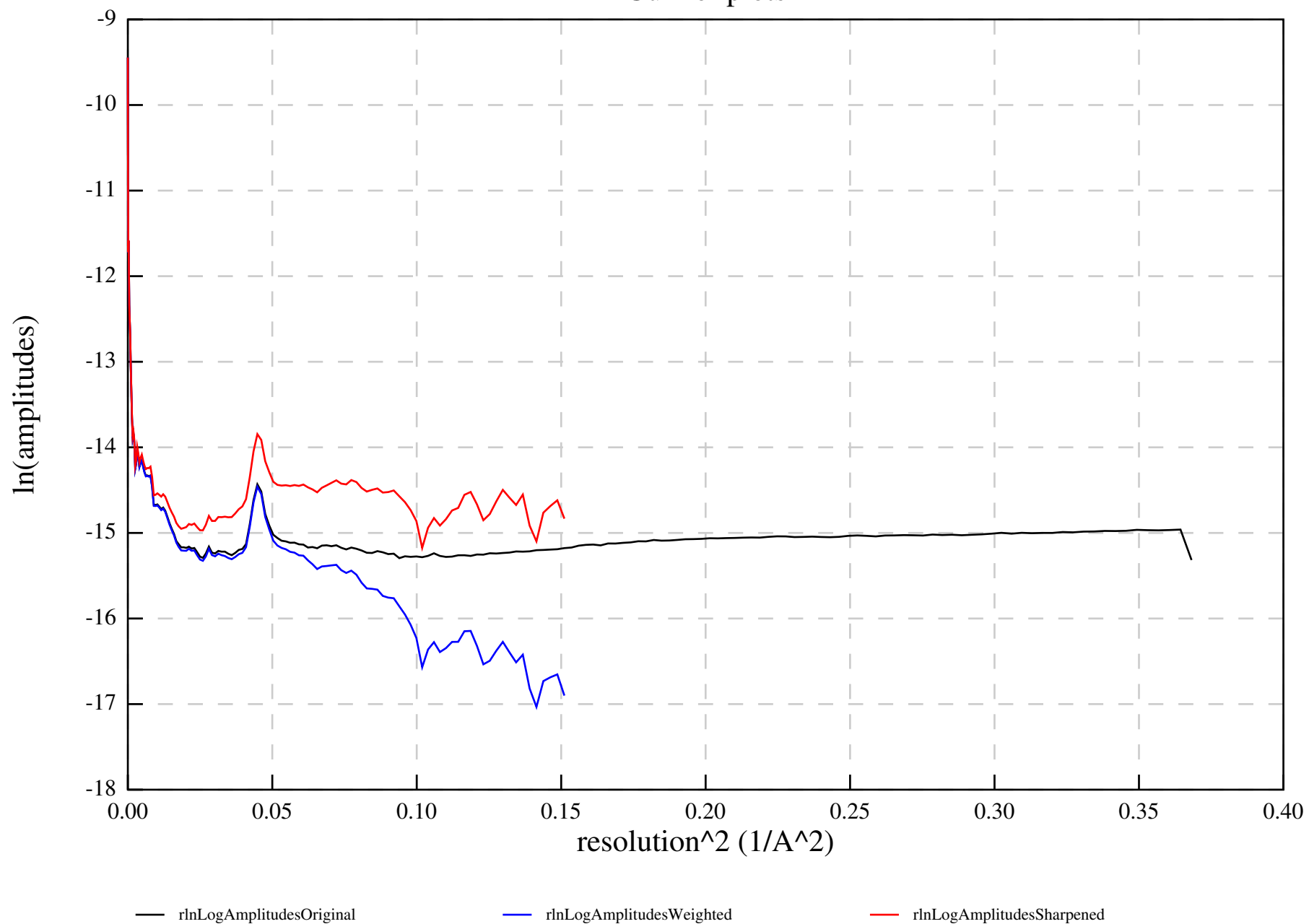
Guinier plots
